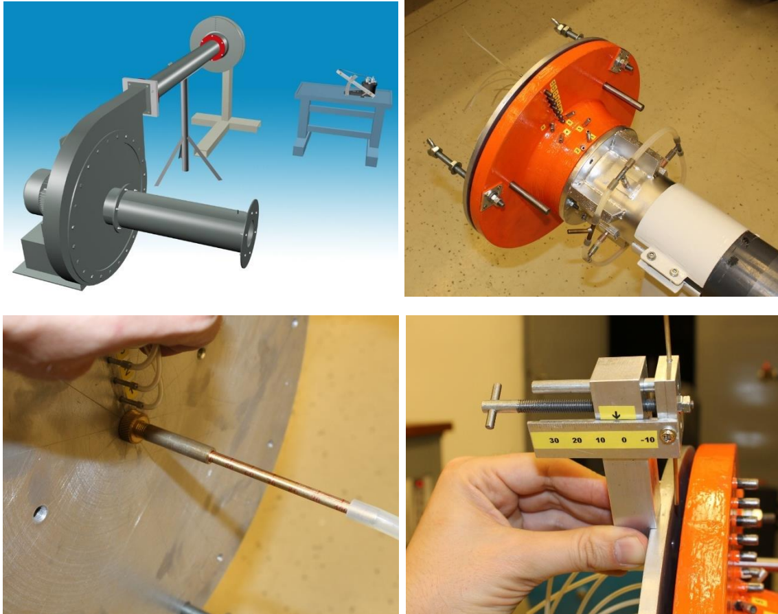
2. ábra. A mérés elrendezése (fent balra); a lapdiffúzor (fent jobbra); statikus nyomás mérése bedugható csővel a középtengelyben (lent balra); sebesség mérése a kilépő keresztmetszetben pozícionálható Pitot-csővel (lent jobbra)
