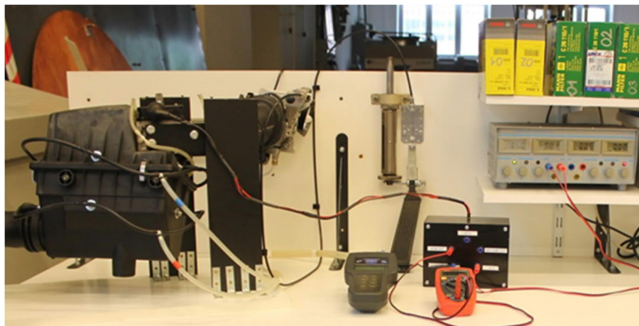
Légszűrő mérőberendezés
