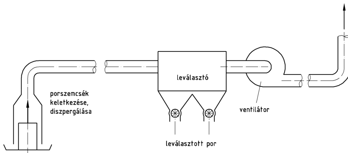
6.1. ábra A portalanító rendszer vázlatát
