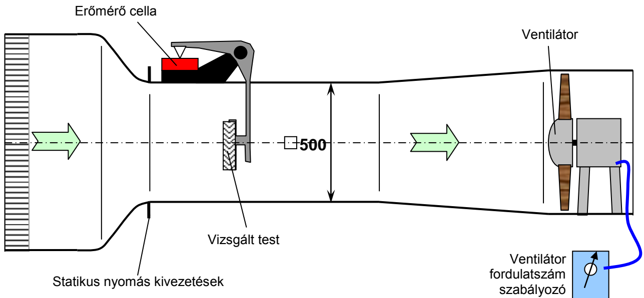
Az NPL típusú szélescsatorna mérési összeállítása
