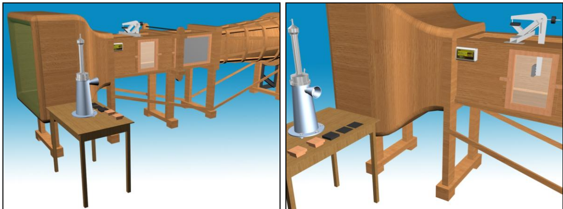
Az NPL típusú szélescsatorna mérési összeállítása
