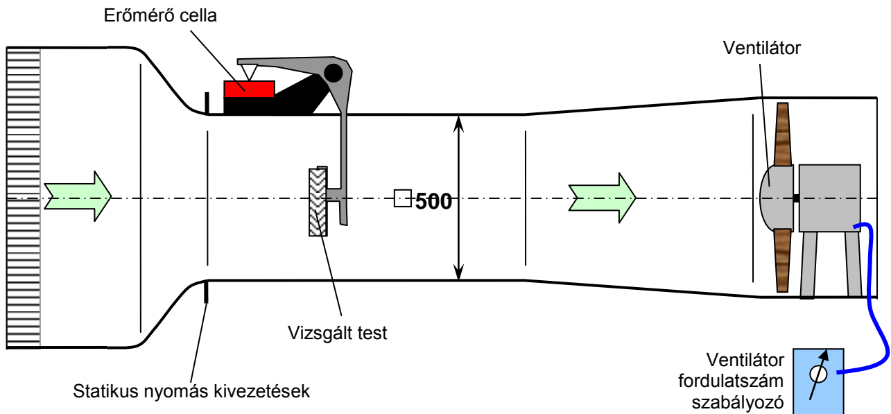
Az NPL típusú szélescsatorna mérési összeállítása
