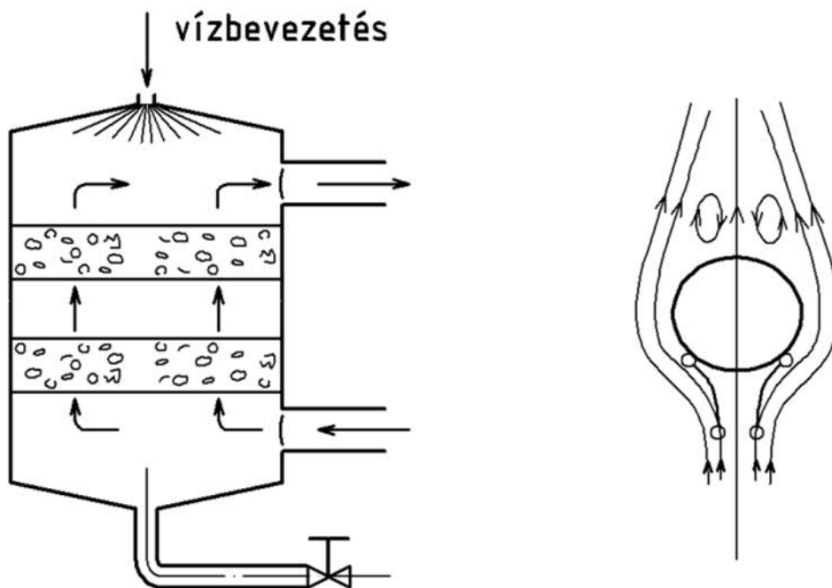
7.7. ábra Mosótorny és egy lefelé hulló vízcsepp körüláramlása
