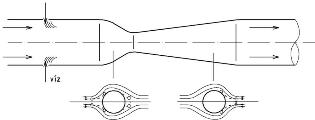
7.8. ábra A Venturi mosó vázlat
