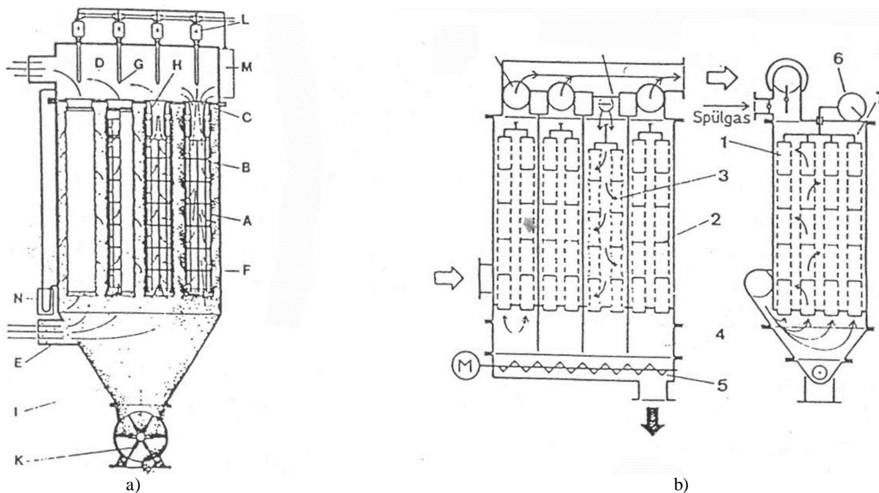
8.15. ábra Zsákos szűrő berendezések (a,b)
