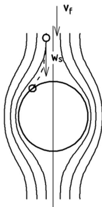
8.4. ábra Felütkezés a súlyerő következtében
