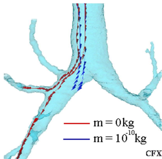
3.4b ábra „Súlytalan” ( m=0\text{kg} , \Psi=0 ) áramlást követő porszemcse (piros vonal) és egy kb. 40 mikron átmérőjű ( m=10^{-10}\text{kg} tömegű, \Psi\approx 250 ) porszemcse (kék vonal) pályák numerikus szimulációval kiszámítva egy hörgő (ld. 1.7 ábra) elágazásban
