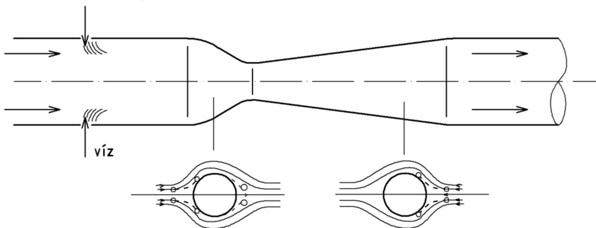
7.8. ábra A Venturi mosó vázolata
