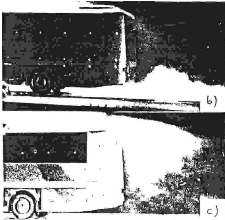
Flow visualisation
